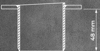
Kołnierz zlicowany z dnem rynny
