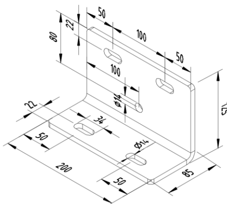
Rysunek 57– Uchwyt przyścienny uniwersalny (możliwe 2 ustawienia).
