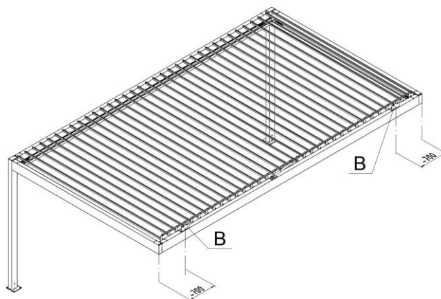
B – Uchwyt ścienny montowany do belki wzdłużnej.
