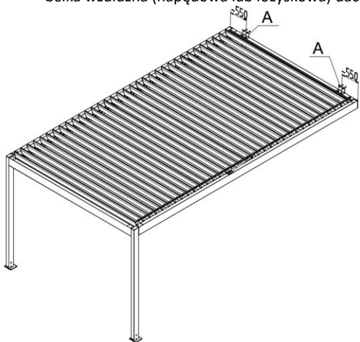
A – Uchwyty ścienne montowane do belek poprzecznych.
